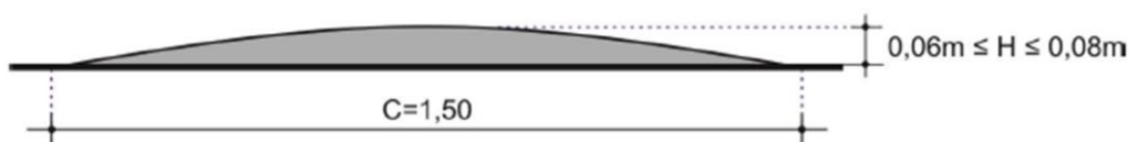
CORTE B-B
