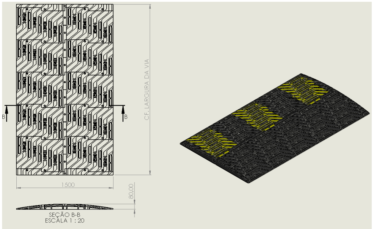
Figura 11 Desenho Montado
